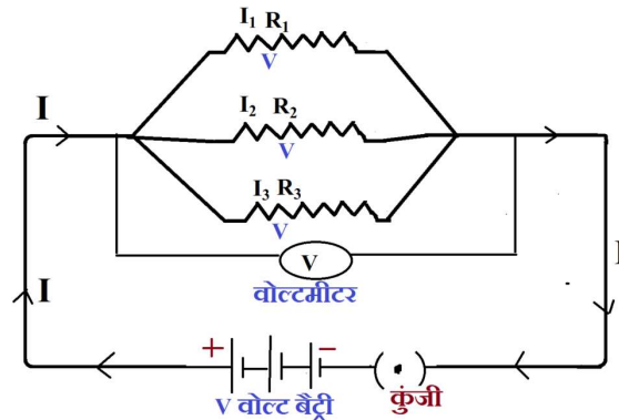
चित्र- विद्युत उपकरणों का समांतर क्रम संयोजन
